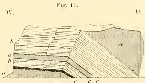
a, a, a Graue Mergel. — b, b Plattige Kalke. — c, c, c Lignitflütze.
