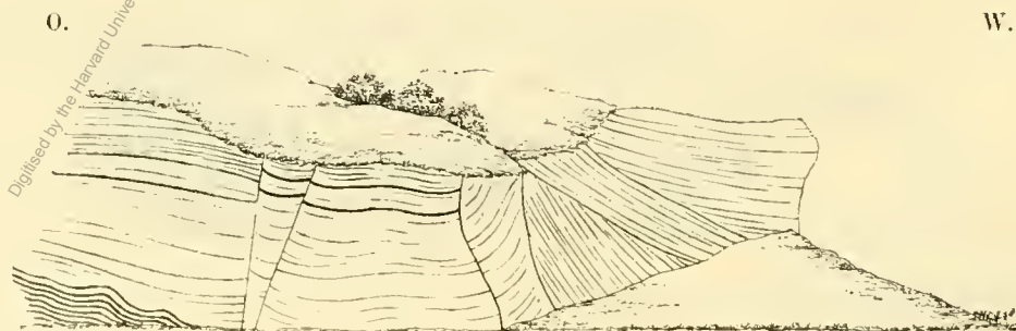
Plattige Kalkbänke mit Verwerfungen.
