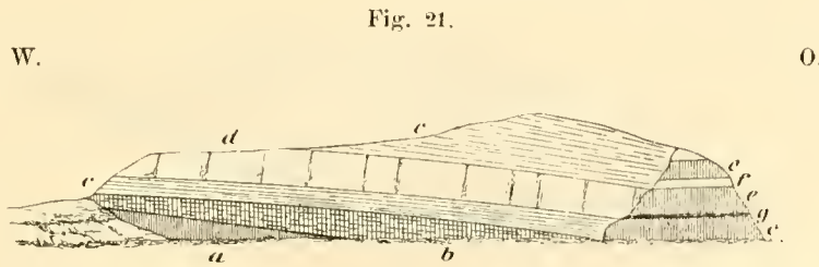
a Blauer Tegel mit kohligen Lignit. — b Travertin. — c Kalkplatten und Mergel. — d Kalkbank. — e Blauer Tegel. — f. Kalkbänke mit Melanopsis und Bithynia . — g Lignit mit Planorbis und Lymnaeus .
