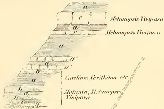
a Graue Mergel. — a' Harte Bänke in den grauen Mergeln. — b Gelbe Mergel, — c Plattige Kalkbänke.
