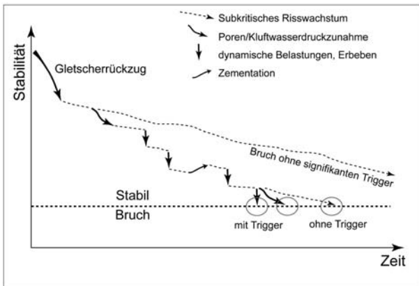
Abb. 37. Schematische Darstellung möglicher Prozesse, die zu einer kontinuierlichen Schwächung des Gesteins führen (subkritisches Risswachstum, Poren/Kluftwasser, Erdbeben). In Gesteinen, in denen Zementationsprozesse in Poren- und Kluft-räumen auftreten (z.B. durch karbonathaltige Wässer), kommt es möglicherweise zu einer Stabilisierung.
