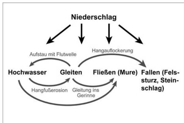
Abb. 38. Mögliche Interaktion von Massenbewegungen, Niederschlag und Hochwasser im alpinen Umfeld.
