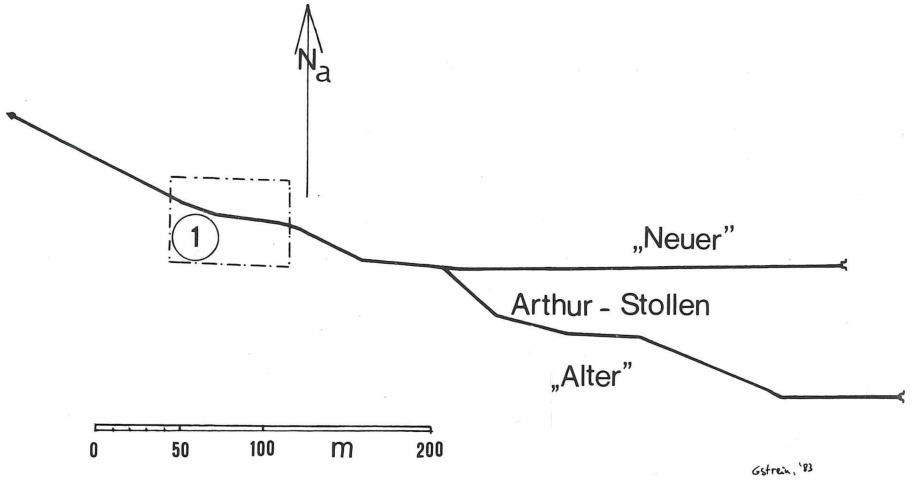
Abb. 1 Übersicht über den Streckenverlauf des östlichsten Teils des Arthur-Stollens. Das ältere Stollenmundloch ist das südlichere, etwas tiefer gelegene. Dieser Stollenteil folgte \pm der Lagerstätte, wobei auf den ersten Meterzehnern durch vorgeschichtliche Baue aufgefahren wurde. Der nördliche Stollenteil wurde erst später, der günstigeren Förderungsbedingungen wegen, geschaffen. – 1 = Der bearbeitete Bereich mit den „Keltenstollen“.
