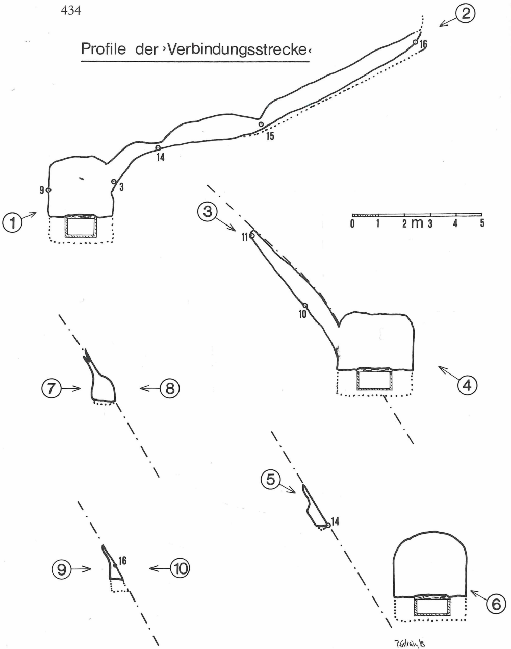
Abb. 5 Profile des ne-lichen Grubenabschnitts („Verbindungsstrecke“).
