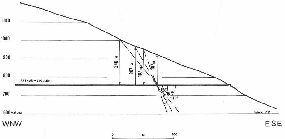
Abb. 7 Längsprofil durch den Westteil des Brander,,ganges“ (Ostabhang des Einödbergs) bzw. den östlichsten Teil des Arthur-Stollens. Eingetragen die Lage der Verschnitte der lagerstättenverwerfenden Scherfläche sowie deren Austrittspunkte am Tag. Daraus Berechnung der Überlagerungshöhe.
