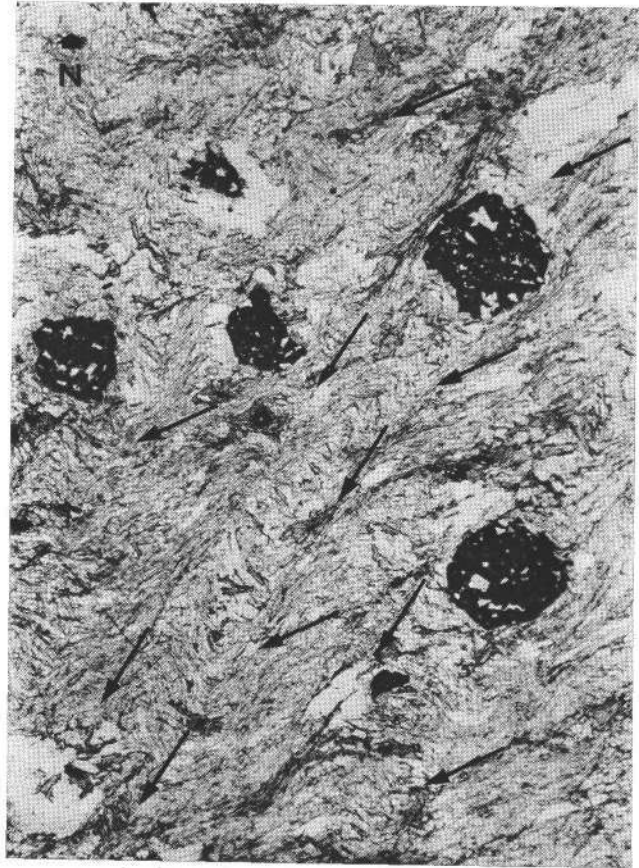
Abb. 4: Dünnschliffaufnahme eines Biotit-Flecken-Gneises mit 15facher Vergrößerung im Hellfeld. Deutlich sind zwei Schieferungen zu erkennen
